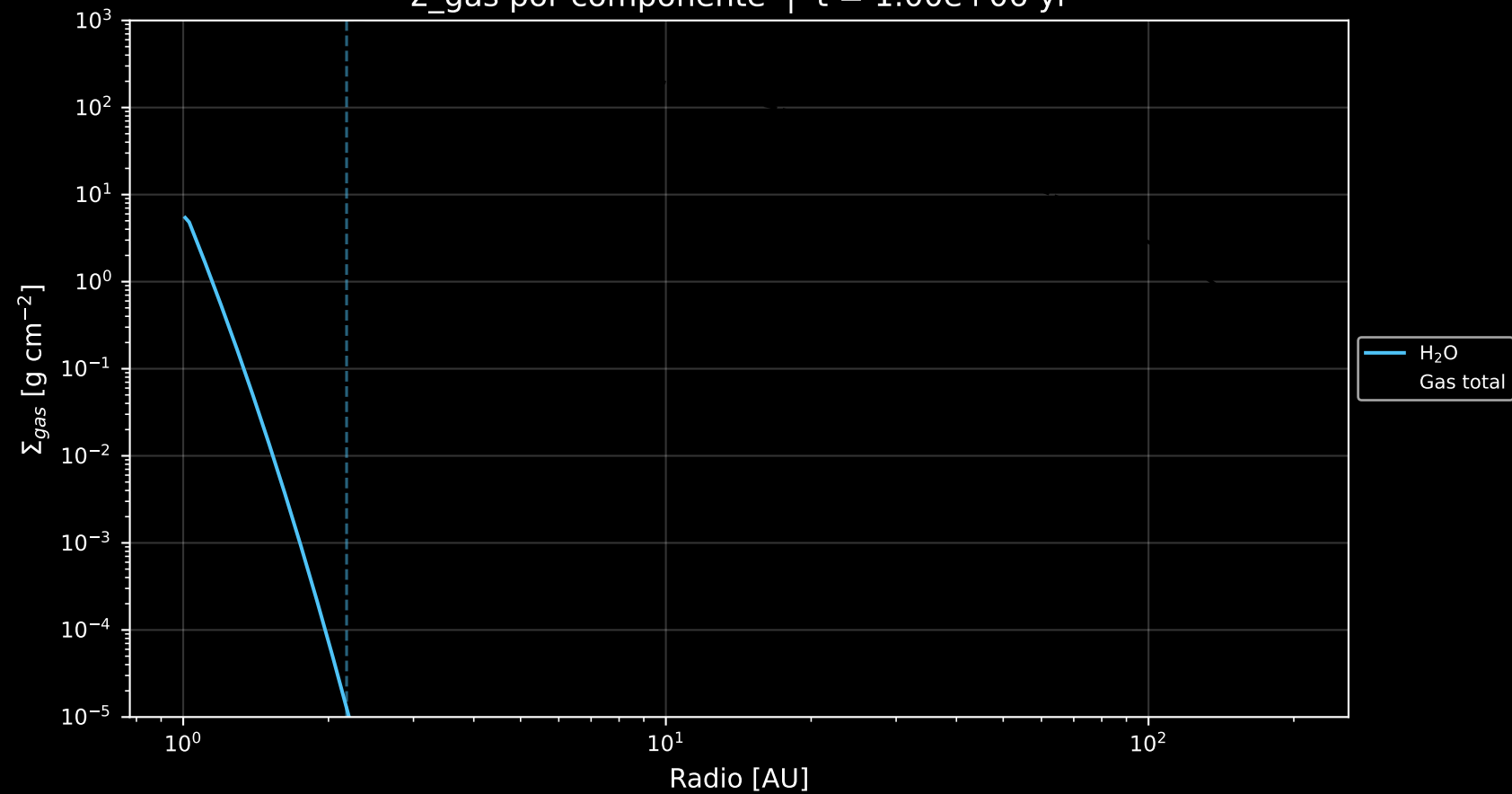
\Sigma_{\text{gas}} por componente | t = 1.00\text{e}+06 yr
